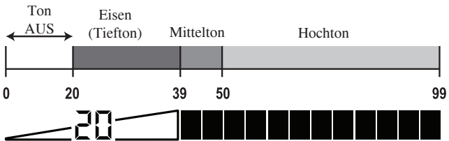
IRON AUDIO AUS: Eisenbereich bis 20 ausgeblendet, Objekte unterhalb von 20 sind nicht mehr hörbar.
